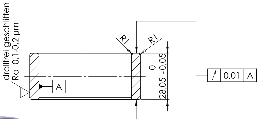
SCHNITT A-A
